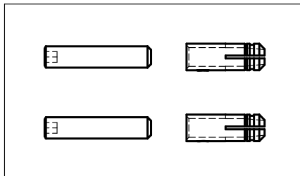
M6 Befestigungsset 266.050.004
